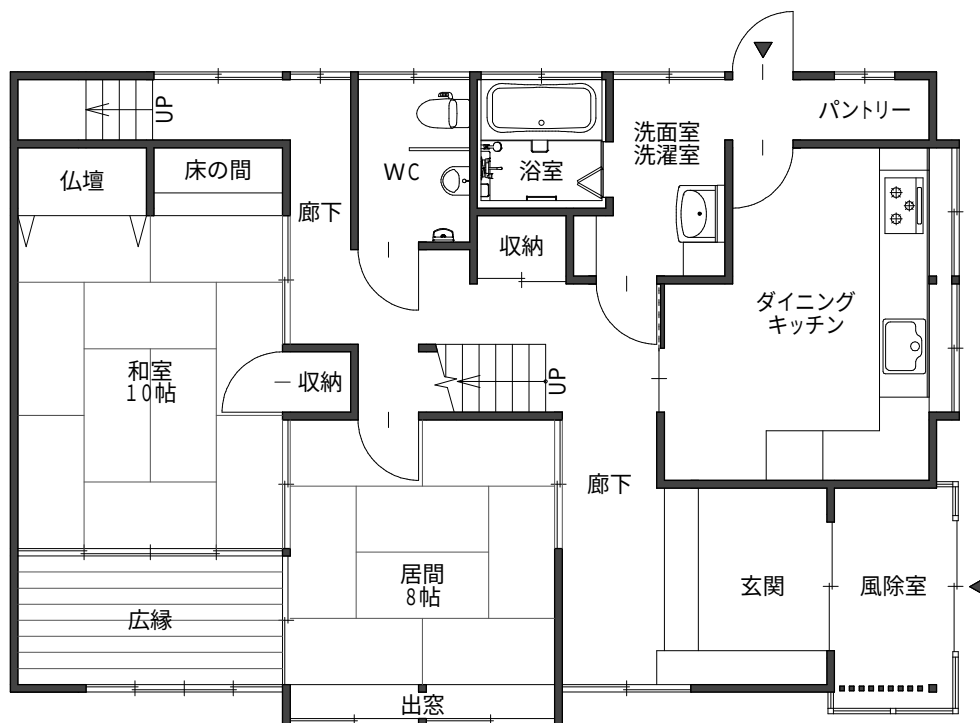
1階平面図
