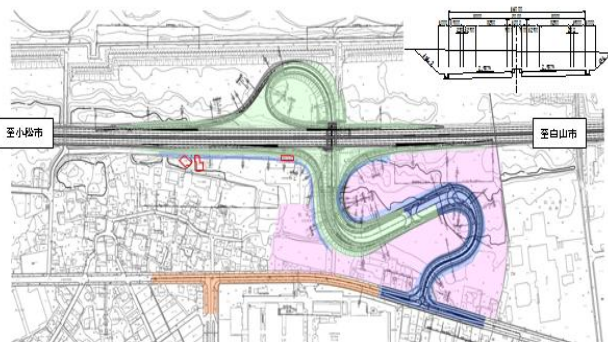
(仮称)能美根上インターチェンジの計画図
