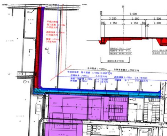
宮竹11号線の計画図
